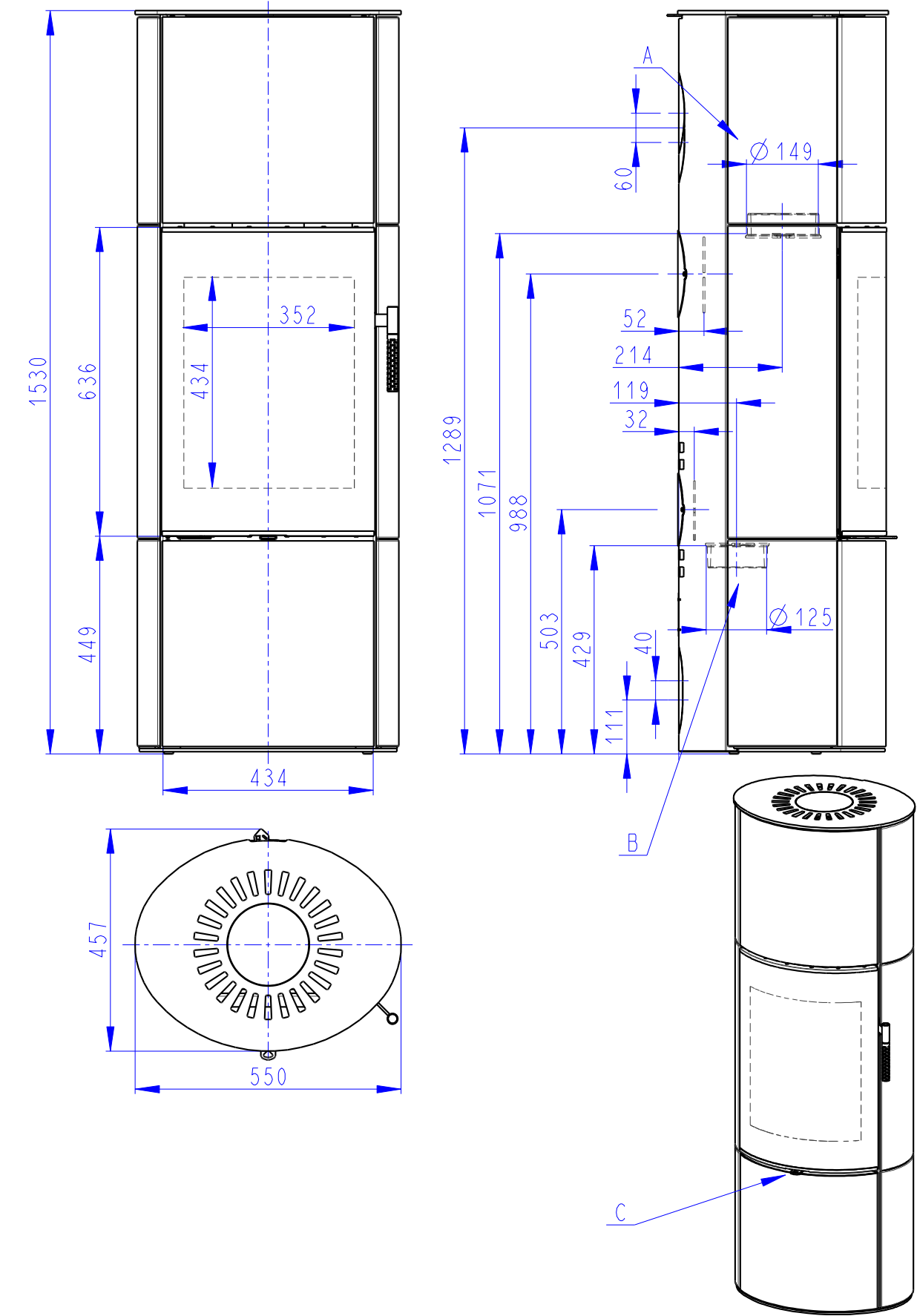
LUGANO 01 A - Dimension sketch, Maßzeichnung, Croquis des dimensions, Dimensioni ingombro
